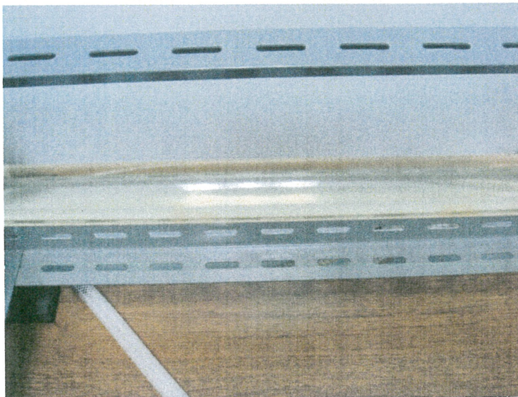
無雑有り5日間循環試験40L/min(左:試験部アクリル配管、右:ホース)
